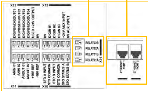
Steuerverdrahtung Anschlüsse AC30V AC30D-P
