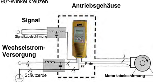
Beispiel AC Fed Inverter gezeigt.
