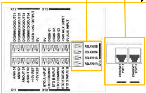
Connessioni cablaggio del sistema (solo AC30D)
