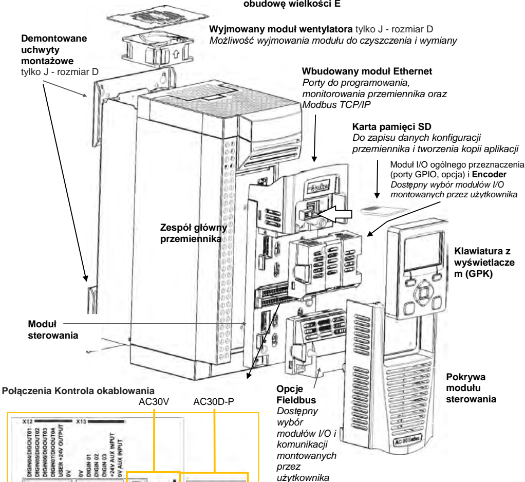
Rysunek przedstawia obudowę wielkości E
