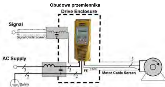
Przykład AC Fed Przetwornica pokazane.
