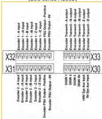
Conexiones de cableado del sistema (Sólo series AC30D)
