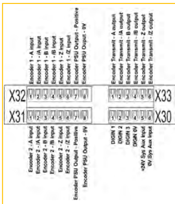
Connessioni cablaggio del sistema (solo AC30D)
